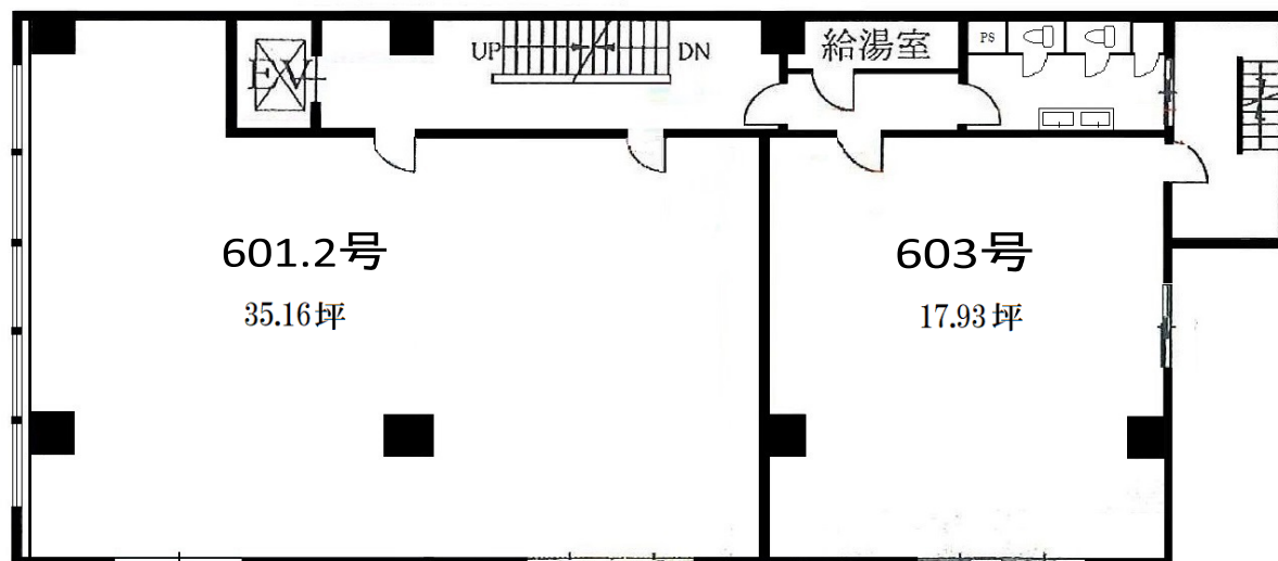
6階平面図
